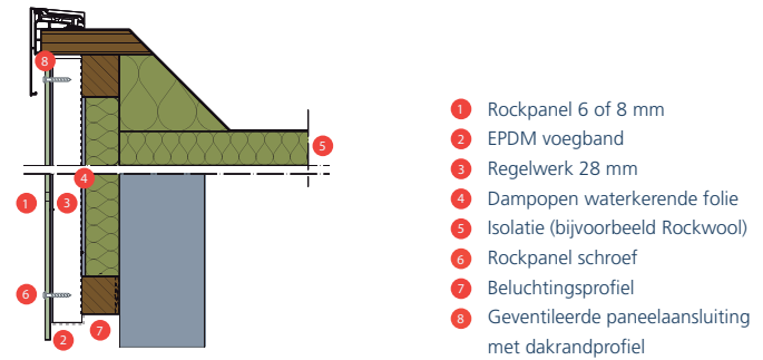
1-501 | mechanische bevestiging op hout, boeiboord nieuwbouw
