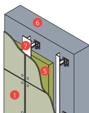
Aluminium draagconstructie
