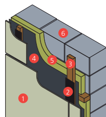
Houten draagconstructie
