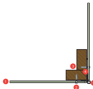
1-208 | mechanische bevestiging op hout, buitenhoek met hoekprofiel
