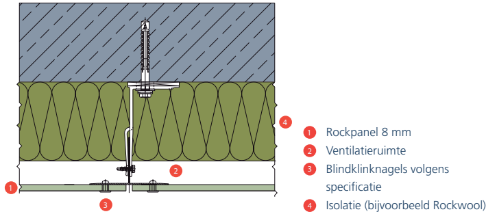
2-200B | mechanische bevestiging op aluminium, plataanluiting
